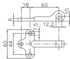
Gegenstück 8 WVG 10-A
