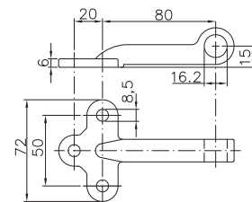
Gegenstück 9 WVG 20-A
