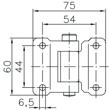
BSCH 30-3
