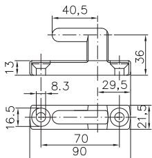
Gegenstück
