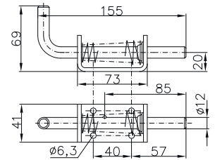
Verriegelungsbolzen BSCHG 20-A
