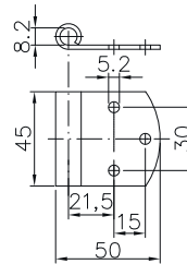
BSCH 50-8-1
