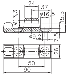
BSCH 40-1
