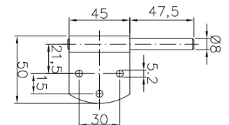
Gegenstück
